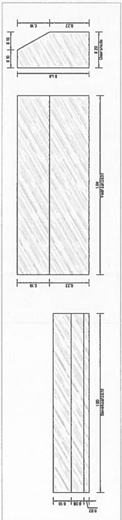
Detail 100/200x400 Busband van natuursteen 1:10
