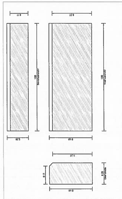
Detail 400x200 opsluitband van natuursteen 1:10
